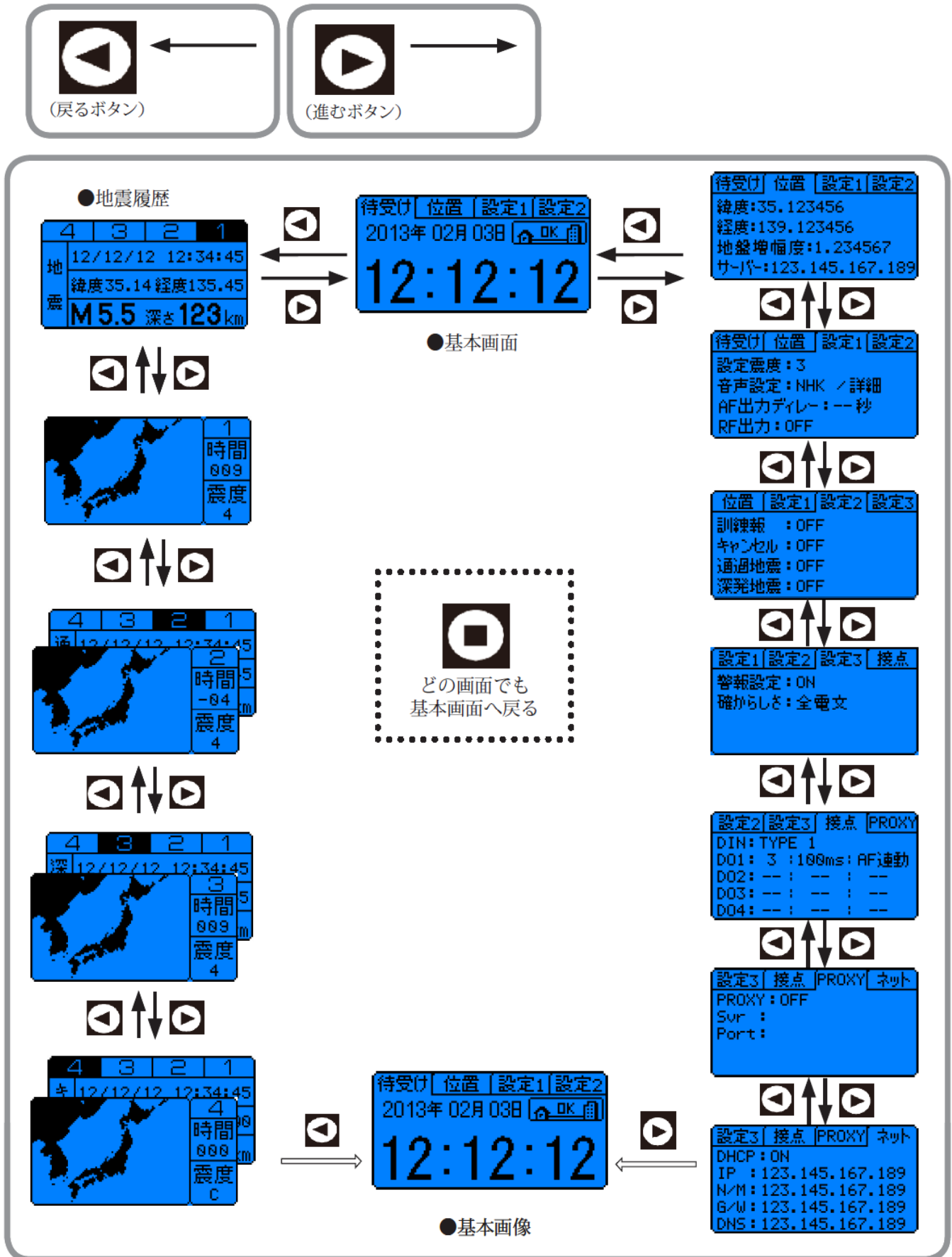
■「地震履歴」 & 「設定情報」の参照操作の画面遷移図
